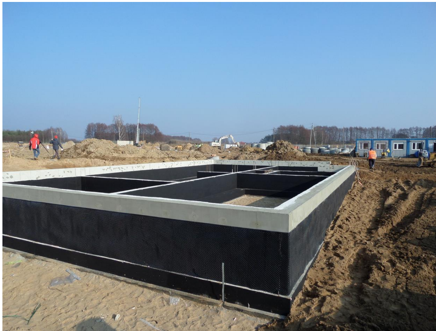
Fundamenty budynku
